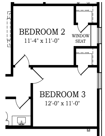
BEDROOM 3 IN LIEU OF GARAGE STORAGE OPTION
